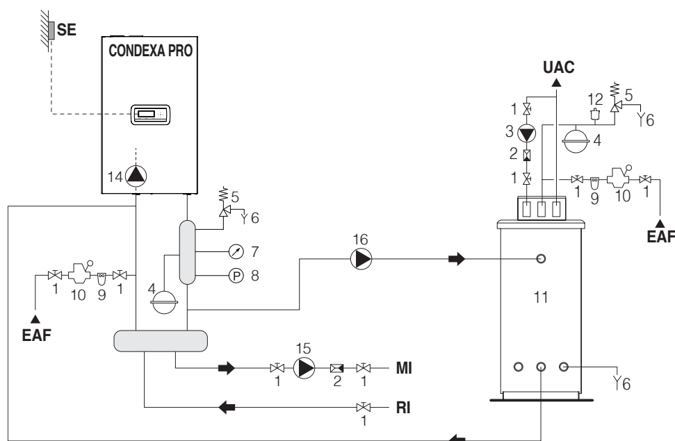
Schemat 4: obieg z kotłem grzewczym podłączonym bezpośrednio do zbiornika c.w.u. oraz za pomocą sprzęgła hydraulicznego do instalacji grzewczej
