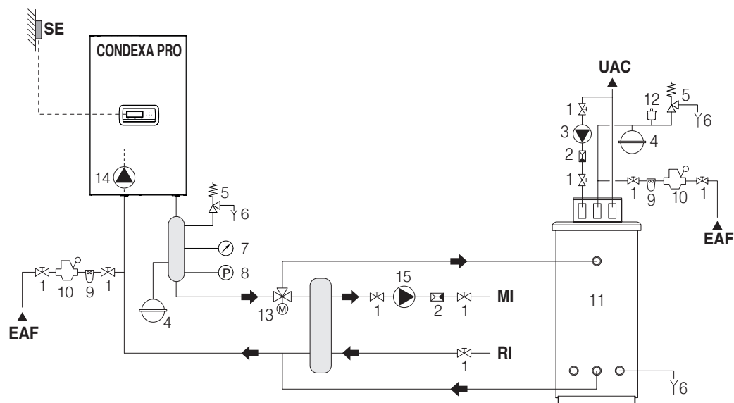
Schemat 5: obieg z kotłem grzewczym podłączonym do instalacji grzewczej i zbiornika c.w.u. za pomocą sprzęgła hydraulicznego
